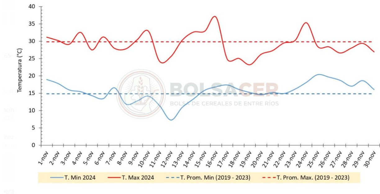
Figura 1: Promedio diario de temperatura mínima y máxima de noviembre del 2024 versus promedio mensual periodo (2019 – 2023).
