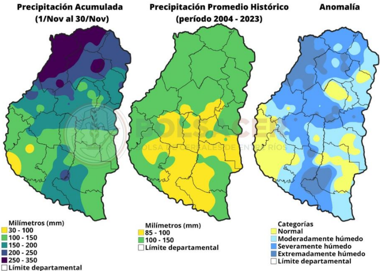
Figura 3 : Distribución espacial de la lluvia acumulada en noviembre de 2024, comparada con el promedio histórico y la anomalía correspondiente
