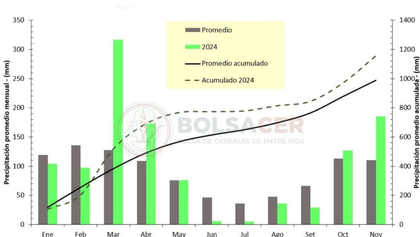
Figura 2 : Comparación de la precipitación promedio mensual y acumulada para noviembre de 2024 con los registros históricos
