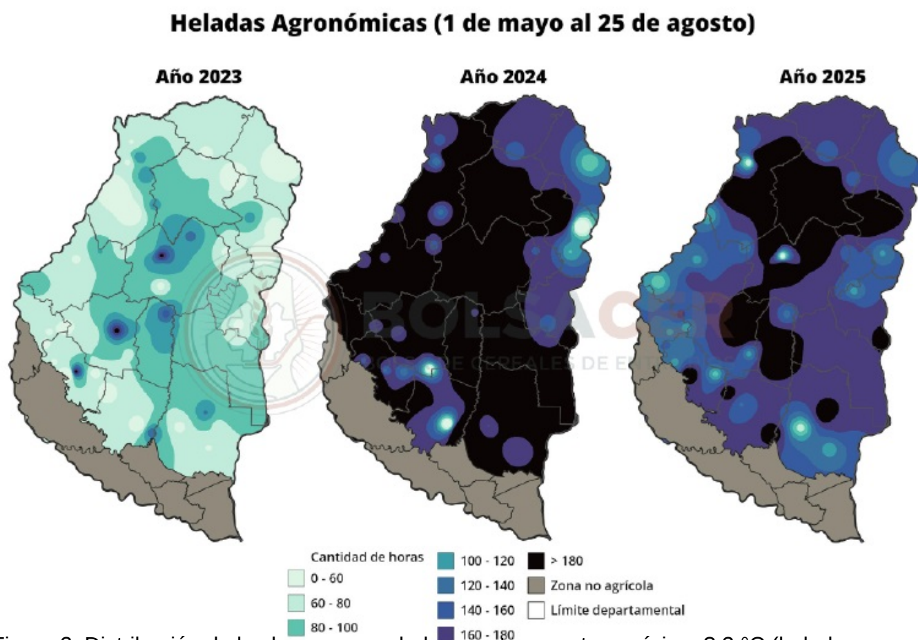
Figura 2: Distribución de las horas acumuladas con temperatura mínima \geq 3 °C (heladas agronómicas) en Entre Ríos, del 01 de mayo al 25 de agosto para los años 2023, 2024 y 2025.
