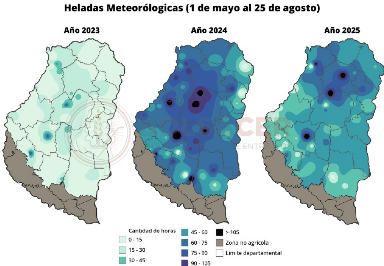
Figura 1: Distribución de las horas acumuladas con temperatura mínima \geq 0 °C (heladas meteorológicas) en Entre Ríos, del 01 de mayo al 25 de agosto para los años 2023, 2024 y 2025.
